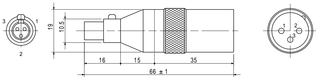
MiXL3-11XLR
