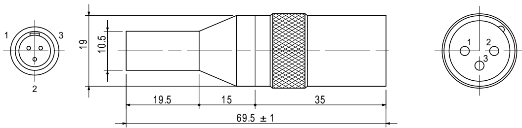
MiXL3-21XLR
