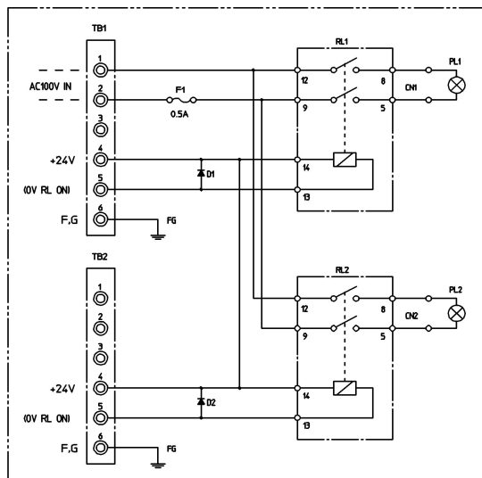
TBX-433回路図
