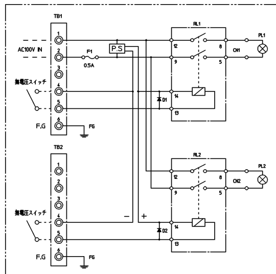
TBX-433P回路図
